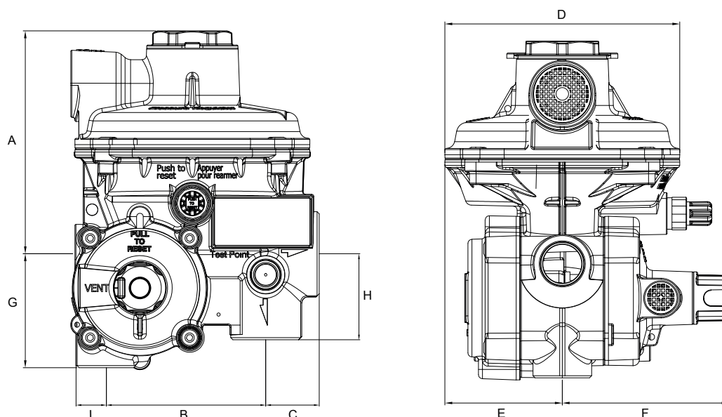
Figura 14 Dimensiones FE25 / FE50
