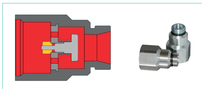
Figura 12 Válvula de seguridad térmica
