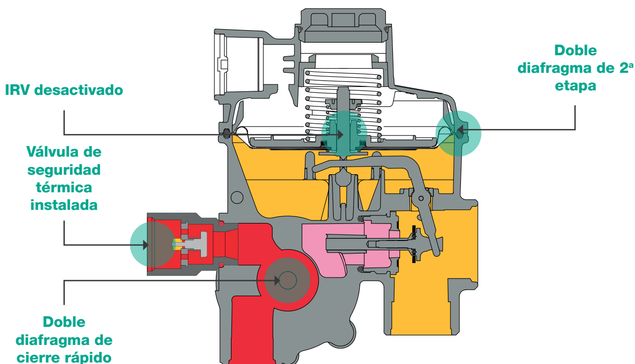
Figura 11 Versión FE NR
