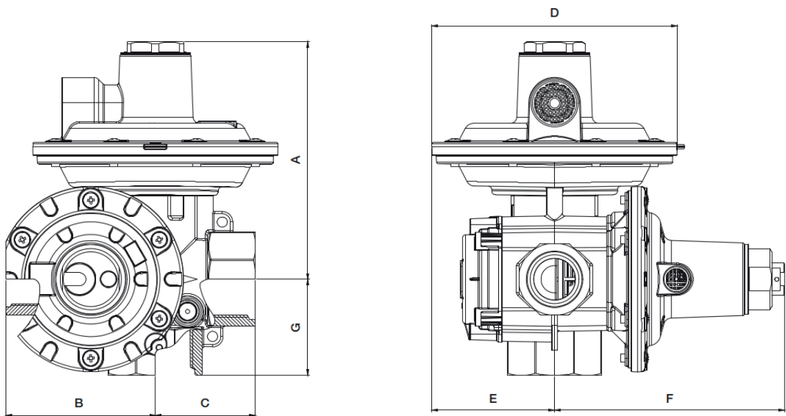
Figura 15 Dimensiones FE75 / FE100
