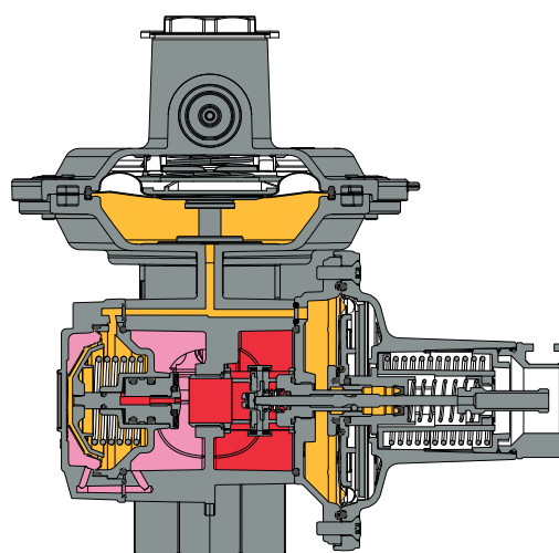
Figura 7 FE75 / FE100 con cierre rápido
