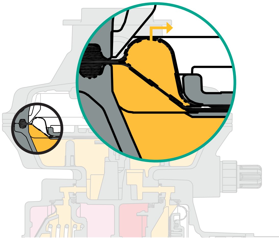
Figura 9 Dobles diafragmas de 2ª etapa
