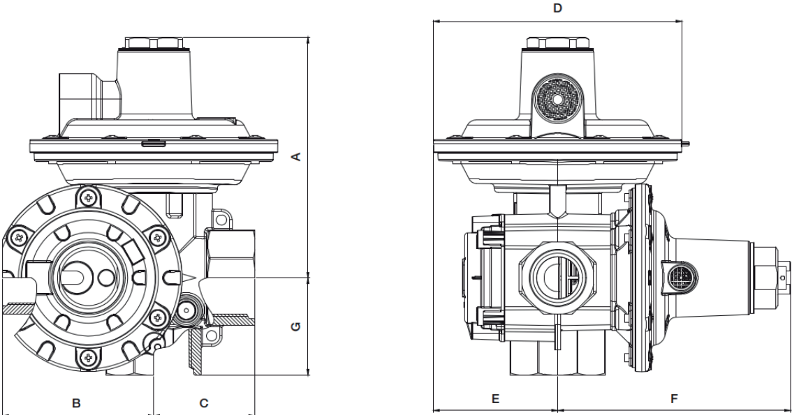
Figure 15 Dimensions de FE75 / FE100
