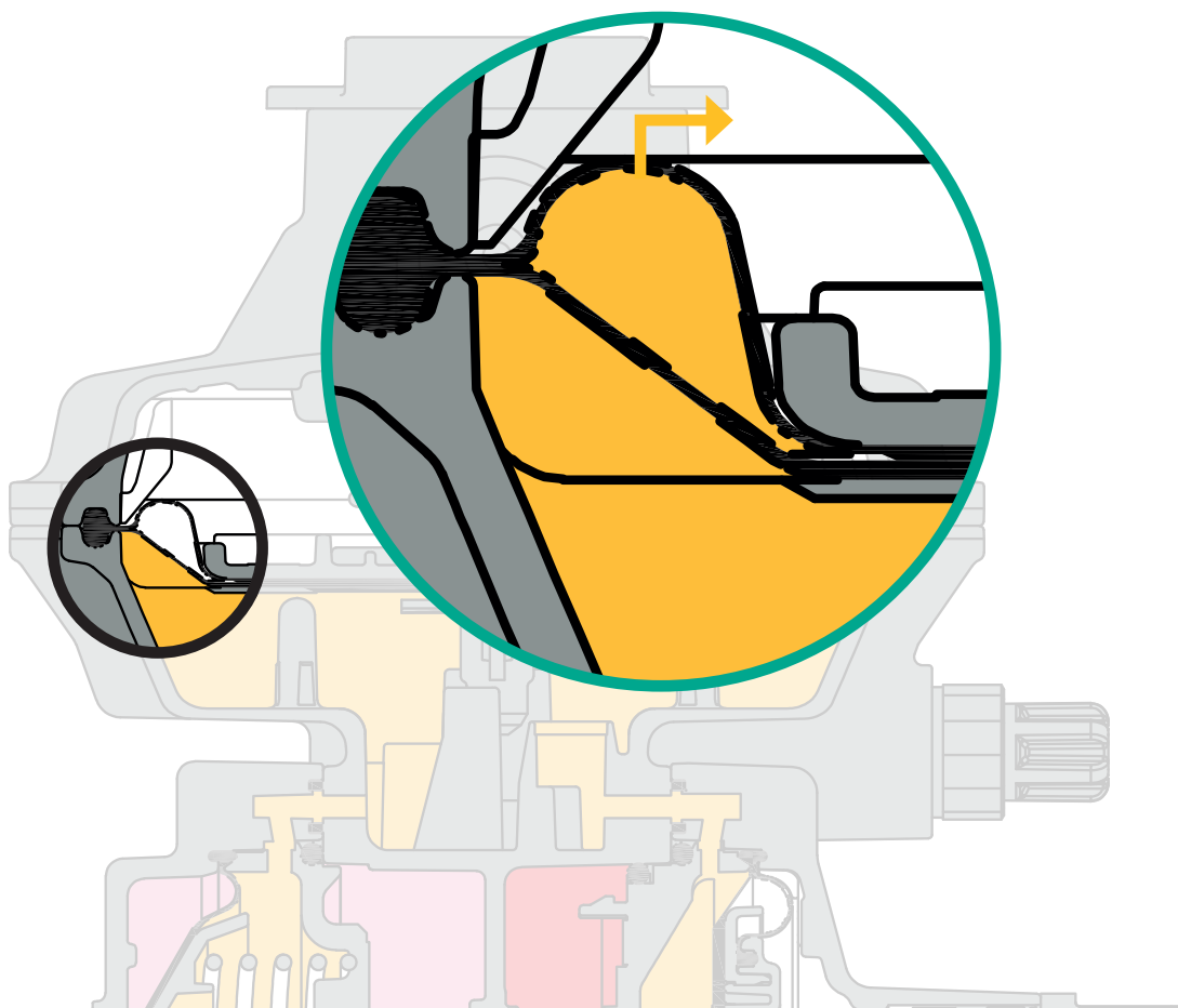
Figure 9 Doubles membranes du 2 e étage du FE
