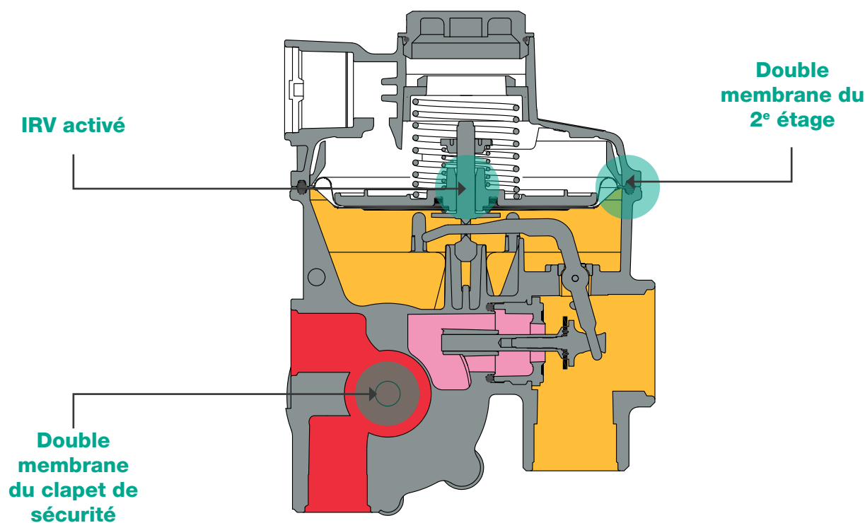
Figure 10 FE en version à évent limité
