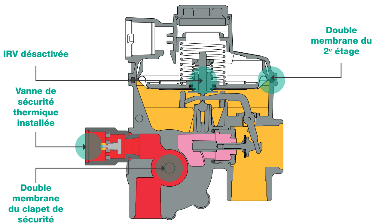
Figure 11 FE en version NR
