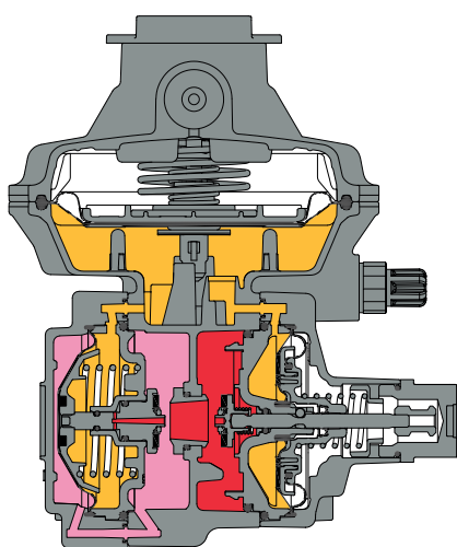
Figure 6 FE25 / FE50 avec clapet de sécurité
